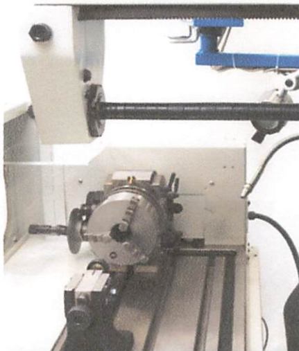
> CABEÇOTE HORIZONTAL E CONJUNTO DIVISOR UNIVERSAL
