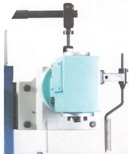
> CABEÇOTE VERTICAL COM SUPORTE ARTICULÁVEL INCORPORADO À MÁQUINA
